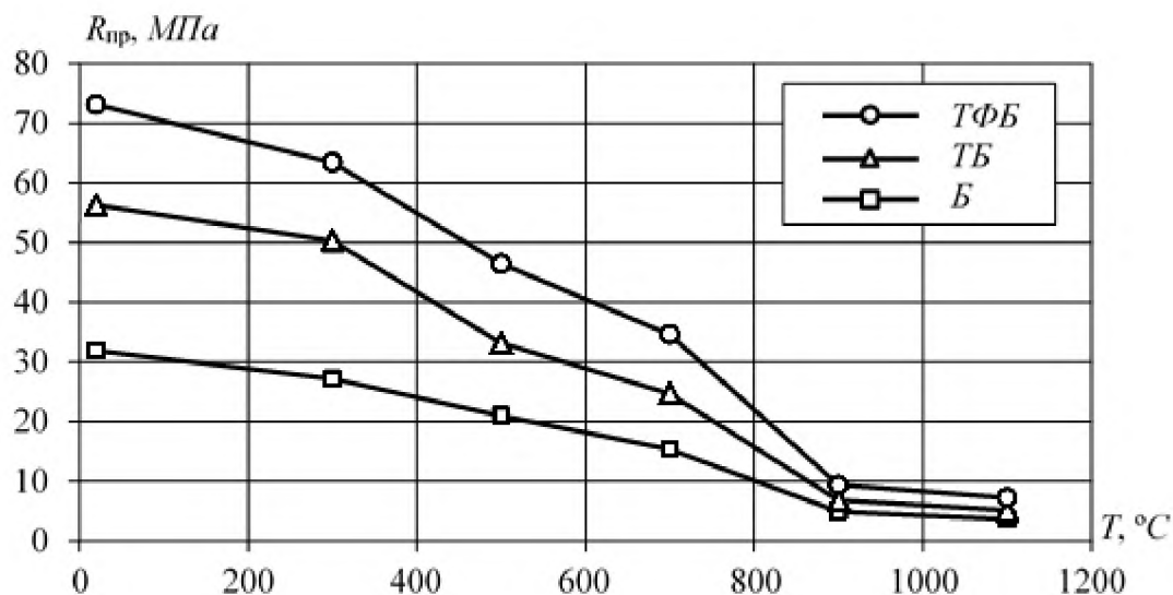
Рис. 1. Экспериментальные зависимости изменения призмочной прочности в образцах бетонов от температуры
