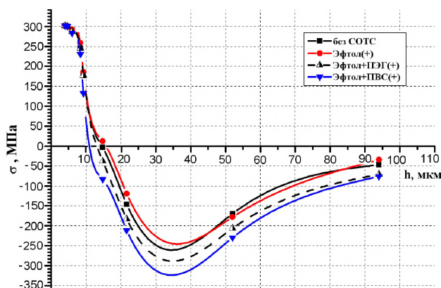
Рис. 4. Остаточные напряжения после точения стали 45 с использованием положительно активированных полимерсодержащих СОТС ( V = 45 м/мин, S = 0,1 мм/об., t = 0,5 мм)
