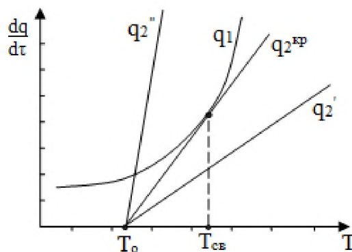
Рис. 2. Соотношение между теплоприходом и теплоотводом:
