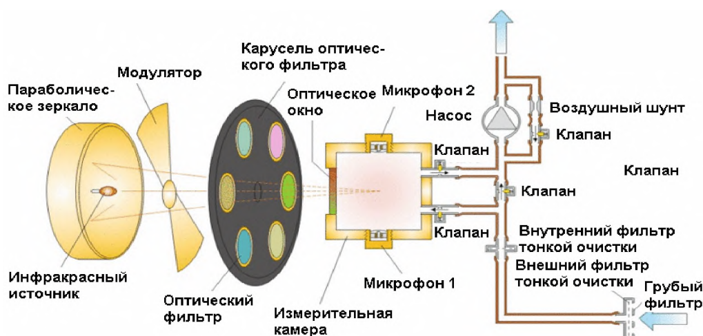
Рис. 1. Структурная схема газоанализатора «Мегакон»
