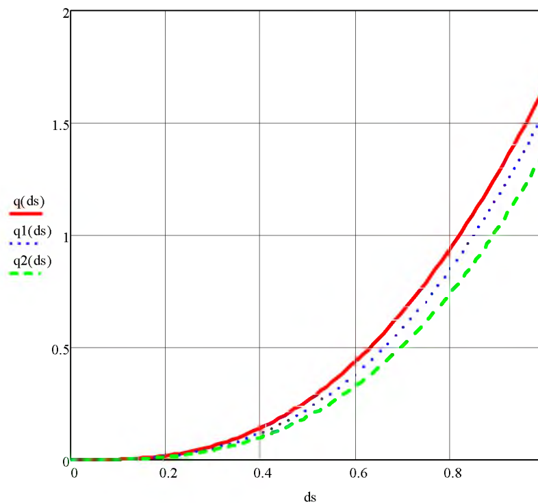
Рис. 3. Зависимость дебита, при котором происходит вынос песка от крупности частиц при разных удельных расходах воздуха: 1–18; 2–25; 3–40 \text{м}^3/\text{м}^3 воды
