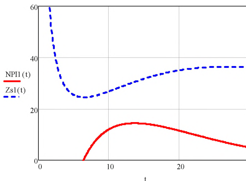
Рис. 2. Динамика среднегодовых величин критериев оптимальности: 1 – чистый приведенный доход NPII(t) , 2 – совокупные дисконтированные затраты Z_s I(t)
